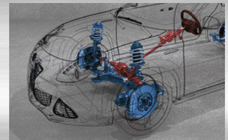
Sicherheitslenksäule
