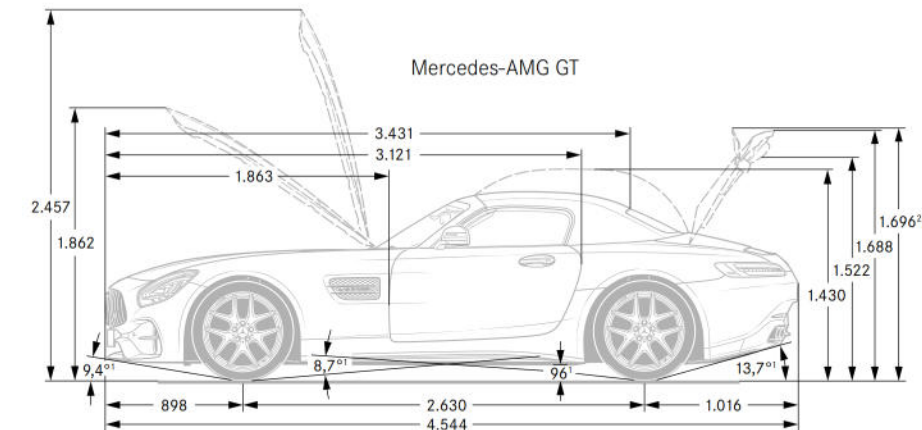
1 Bei zulässigem Gesamtgewicht 2 Spoiler ausgefahren Maße Mercedes-AMG GT S geringfügig abweichend
