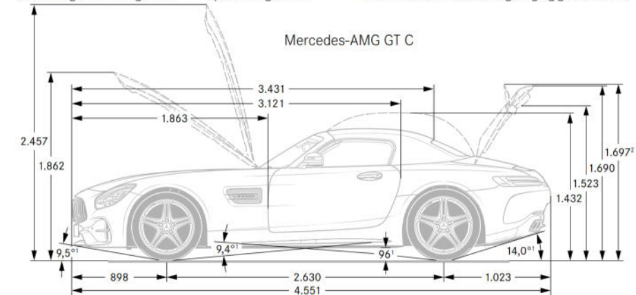
1 Bei zulässigem Gesamtgewicht 2 Bei ausgefahrenem Heckspoiler 3 In Anlehnung an Richtlinie ISO 3832:2002-06. Gepäckraumvolumen kann je nach Sonderausstattung abweichen
