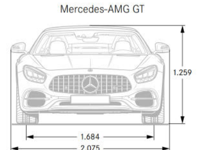
Maße Mercedes-AMG GT S geringfügig abweichend
