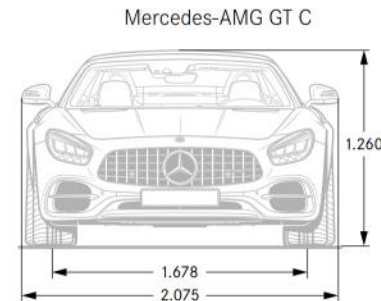
1 Bei zulässigem Gesamtgewicht 2 Bei ausgefahrenem Heckspoiler 3 In Anlehnung an Richtlinie ISO 3832:2002-06. Gepäckraumvolumen kann je nach Sonderausstattung abweichen
