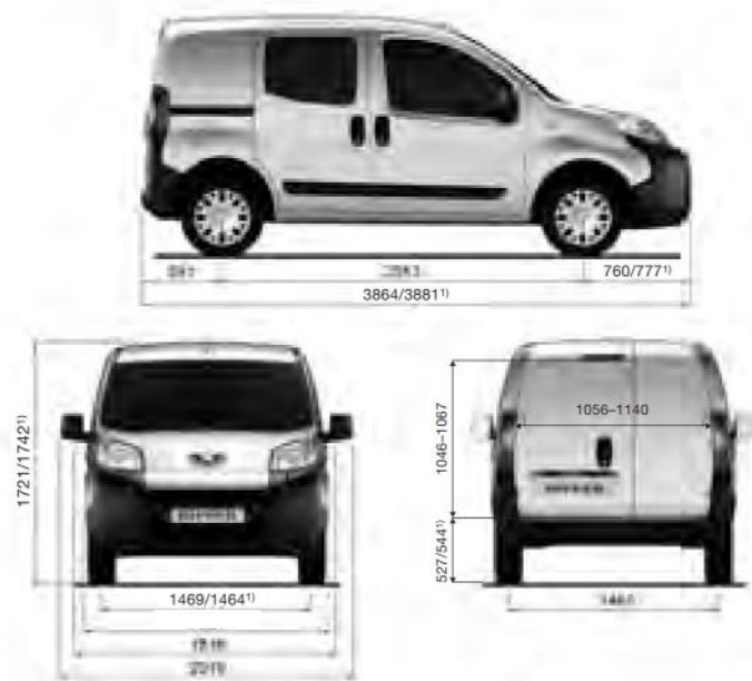
Höhe mit Dachreling (mm): 1782/1803 1)
